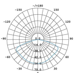
Beam angle: 148°
